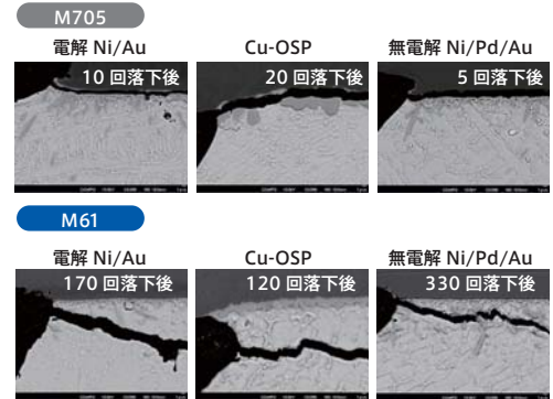
M705 は接合界面、M61 ははんだバルクで破断
