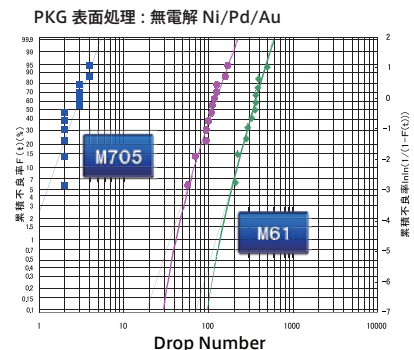
M705 は接合界面、M61 ははんだバルクで破断
