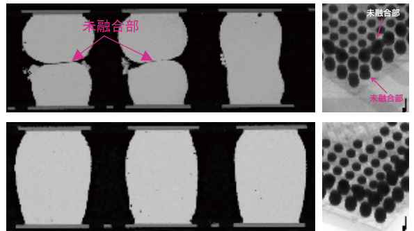
良好な転写性を示す NSV320
