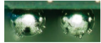
転写性が欠如する印刷用ペースト
