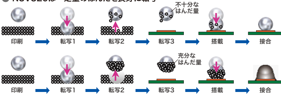
転写性が欠如する印刷用ペースト
